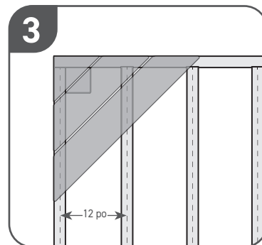
3 INSTALLATION DE L'INFRASTRUCTURE DIAGONALE
