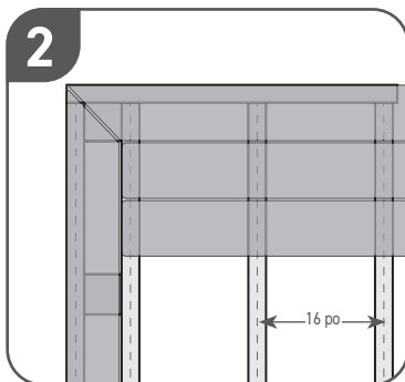
2 INSTALLATION DE L'INFRASTRUCTURE D'ENCADREMENT
